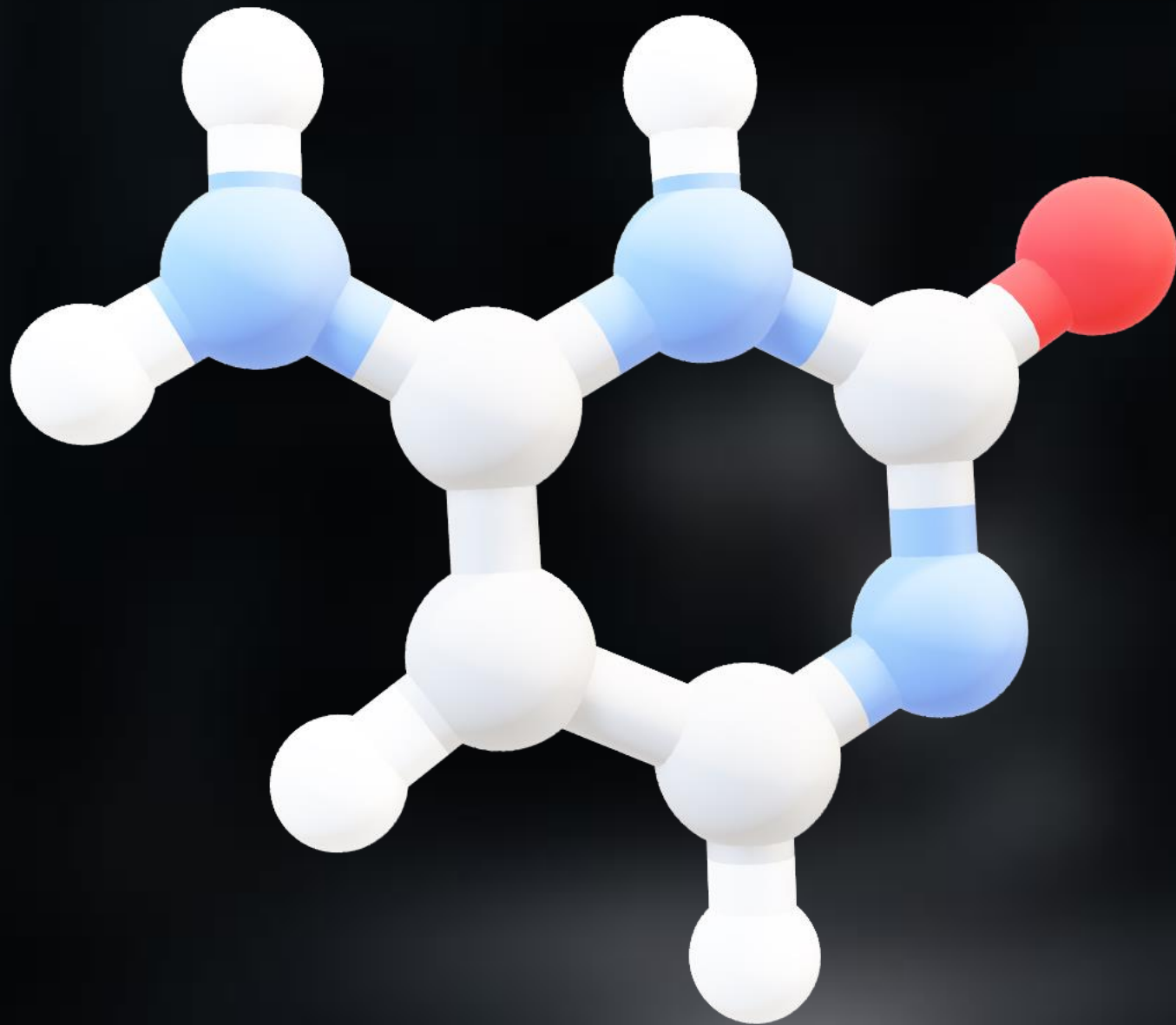
Cytosine
