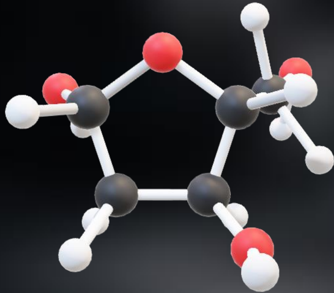
Deoxyribose
